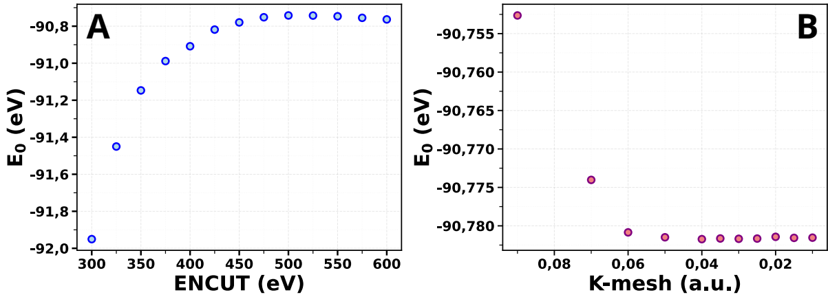
Figura 4: Gráfico de convergência da energia total do sistema em função dos parâmetros ENCUT e k -points.
